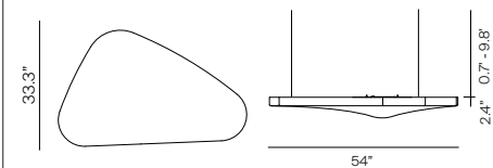
D71 PD canopy Ø 4.5" x h 1.2"
