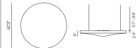
D71 CD canopy Ø 4.5" x h 1.2"
