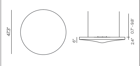
D71 CD canopy Ø 4.5" x h 1.2"
